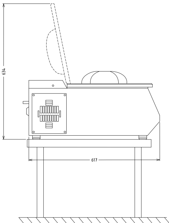
Zij aanzicht
