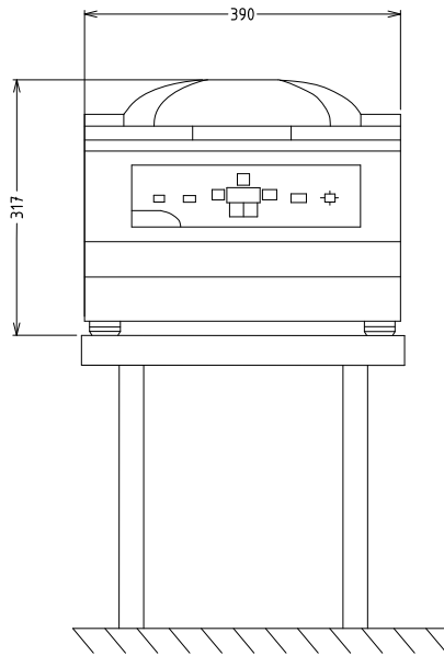
Front aanzicht
